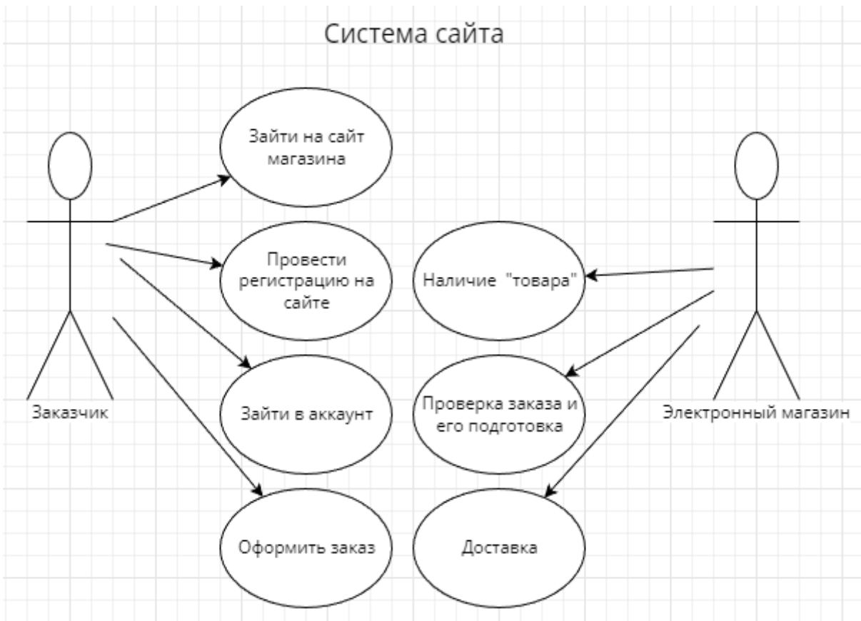
Рисунок 1.2 Диаграмма вариантов использования “Электронный магазин”
