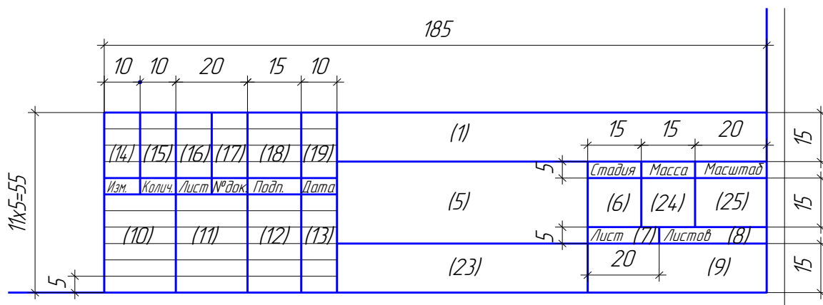
Рисунок 24 – Основная надпись для документации для строительства
