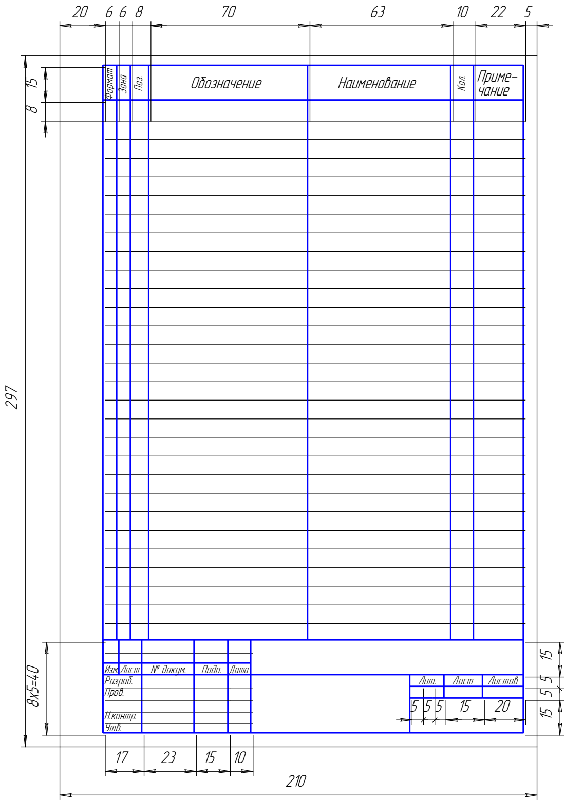
Рисунок К.4 – Спецификация
