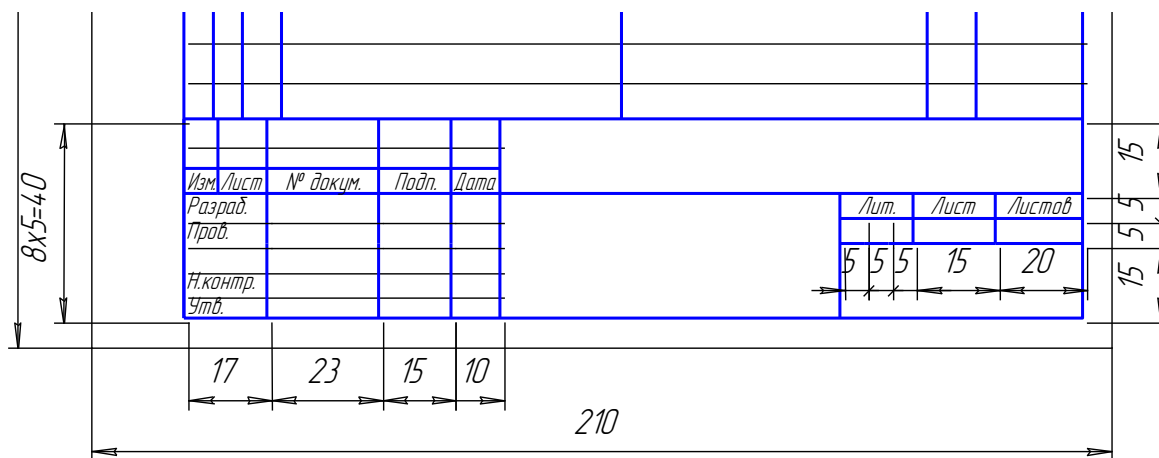
Рисунок 22 – Основная надпись для спецификаций (первый лист)
