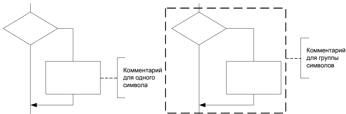
Рисунок 9 – Использование комментария
