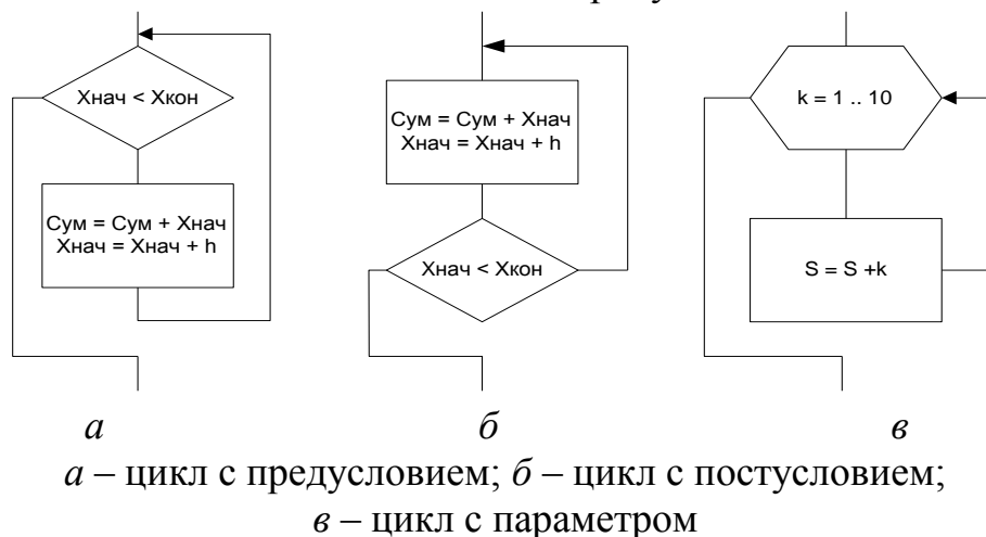
Рисунок 16 – Изображение циклов
