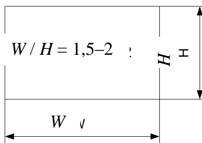
Рисунок 8 – Размеры символов
