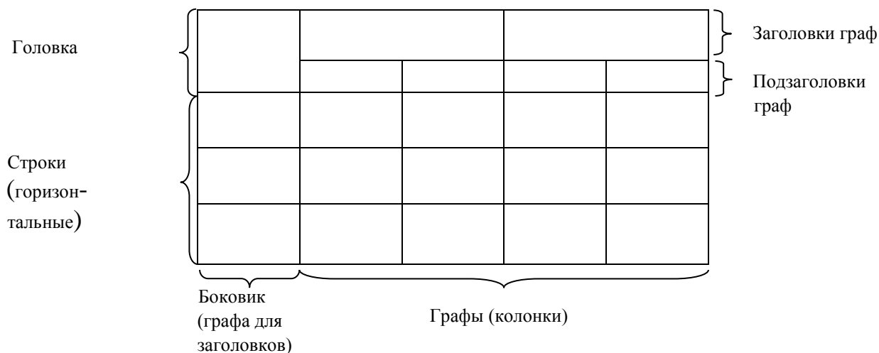
Рисунок 7 – Элементы таблицы
