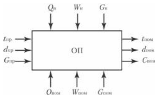
Рис. 5 Обобщенная функциональная модель обслуживаемого помещения (ОП) как объекта регулирования
