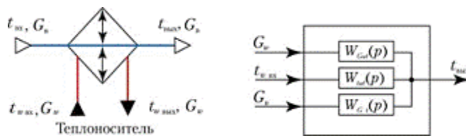
Рис. 7 Функциональная и структурная схемы теплообменника типа «жидкость-воздух»
