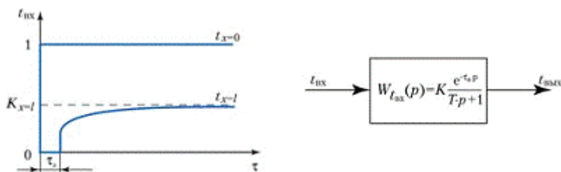
Рис. 10 Характеристика воздуховода как объекта управления: а - переходной процесс изменения температуры; б - передаточная функция
