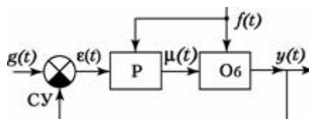
Рис. 3 Обобщенная структурная схема САР: Об - объект регулирования с передаточной функцией W_{Об}(p) ; СУ - устройство сравнения; P - регулятор с передаточной функцией W_p(p) ; f(t) - возмущающее воздействие; y(t) - регулируемая величина; \varepsilon(t) - ошибка регулирования g(t) - задающее воздействие; \mu(t) - управляющее воздействие
