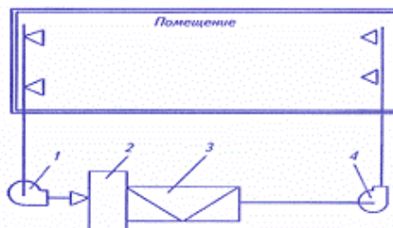
Рис. 1. Принципиальная схема центральной рециркуляционной (замкнутой) СКВ: 1 - вытяжной вентилятор; 2 - воздухоприемная камера; 3 - центральный кондиционер; 4 - приточный вентилятор
