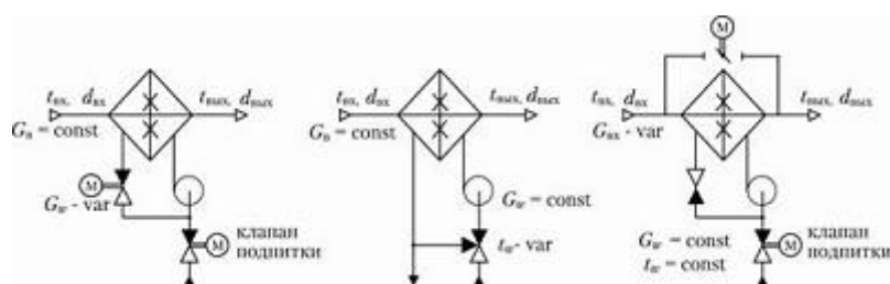
Рис. 9 Методы управления оросительной камерой: а - расходом жидкости; б - температурой теплоносителя; в - расходом воздуха
