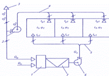
Рис. 2. Принципиальная схема однозональной центральной СКВ с частичной рециркуляцией: 1 - воздухоприемная камера; 2 - вытяжной вентилятор; 3 - воздуховыбросная шахта; 4 - воздуховод вытяжной системы; 5 - приточный воздуховод; 6 - вентилятор; 7 - центральный кондиционер
