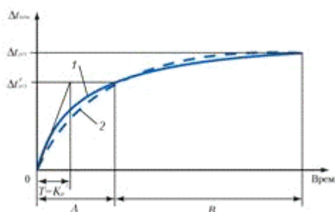
Рис. 6 Процесс изменения температуры в помещении: 1 - эксперимент; 2 – расчет
