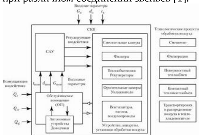
Рис. 4. Обобщенная структурная схема СКВ как объекта автоматизации: t_n , d_n , G_n - температура, влажность, расход наружного воздуха; t_{пом} , d_{пом} , G_{пом} - температура, влажность, расход воздуха в помещении; Q_t , Q_w , Q_g - тепловая, влажностная и газовые нагрузки
