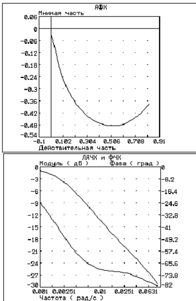
Рис 12. ЛАЧ и ЛФЧ при астатическом регулировании.
