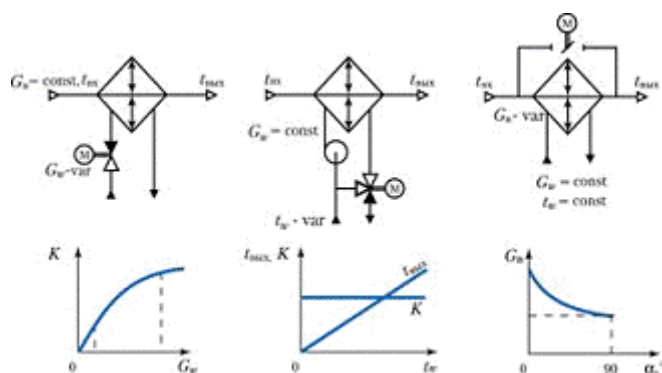
Рис. 8 Способы управления поверхностными теплообменниками типа «жидкость-воздух»: а - расходом жидкости; б - температурой теплоносителя; в - расходом воздуха
