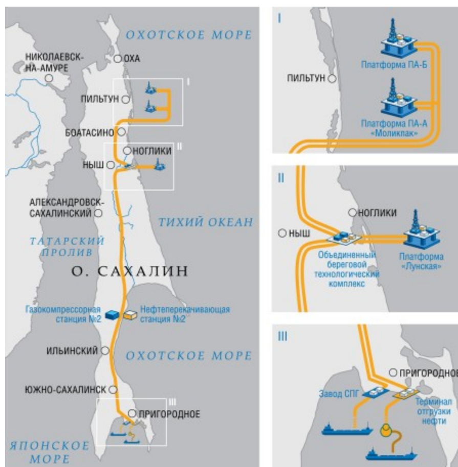
Рисунок 5. Проект "Сахалин-2"
