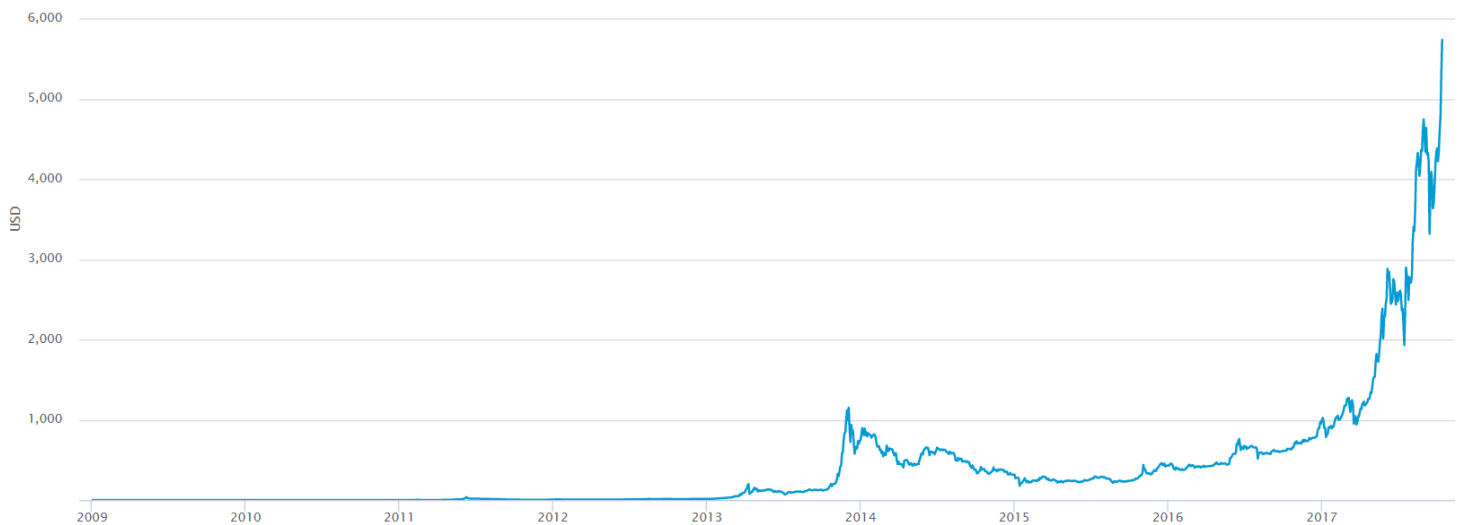
Рисунок 2 График роста курса биткоина
