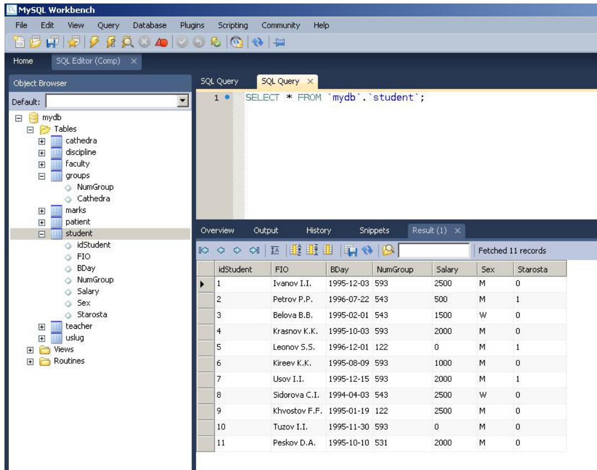
Рис. 2.8 – MySQL Workbench 5.2
