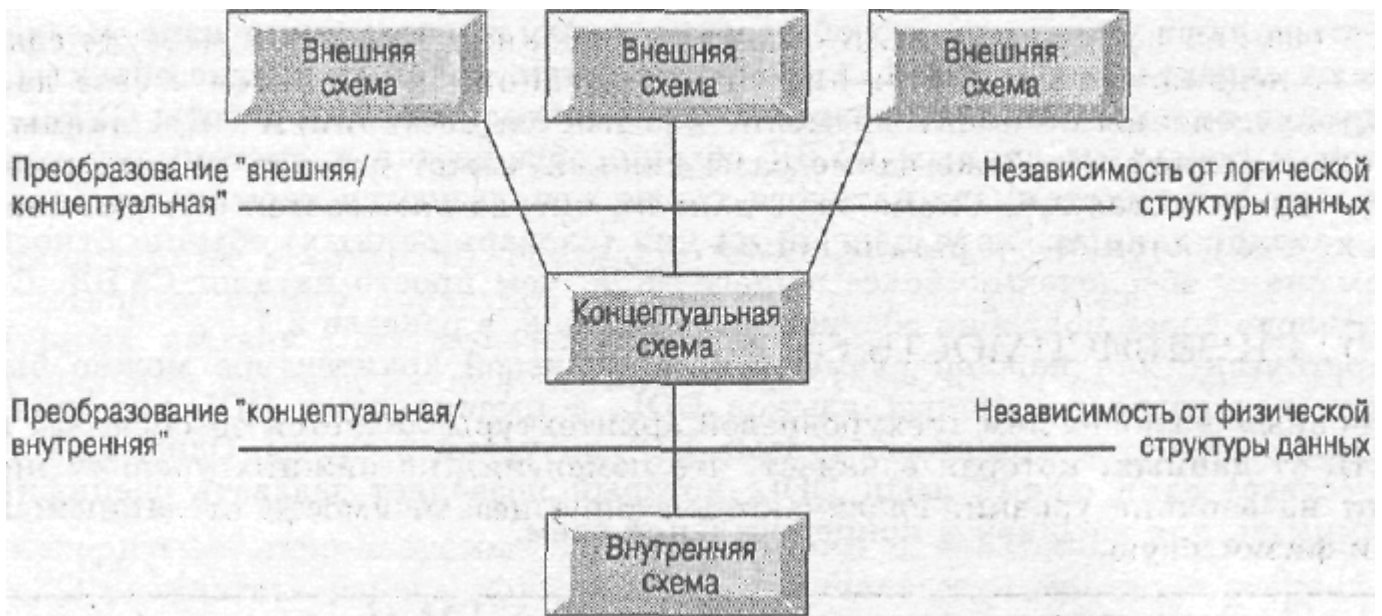
рисунок 2. Реализация независимости от данных в трехуровневой архитектуре ANSI-SPARC.
