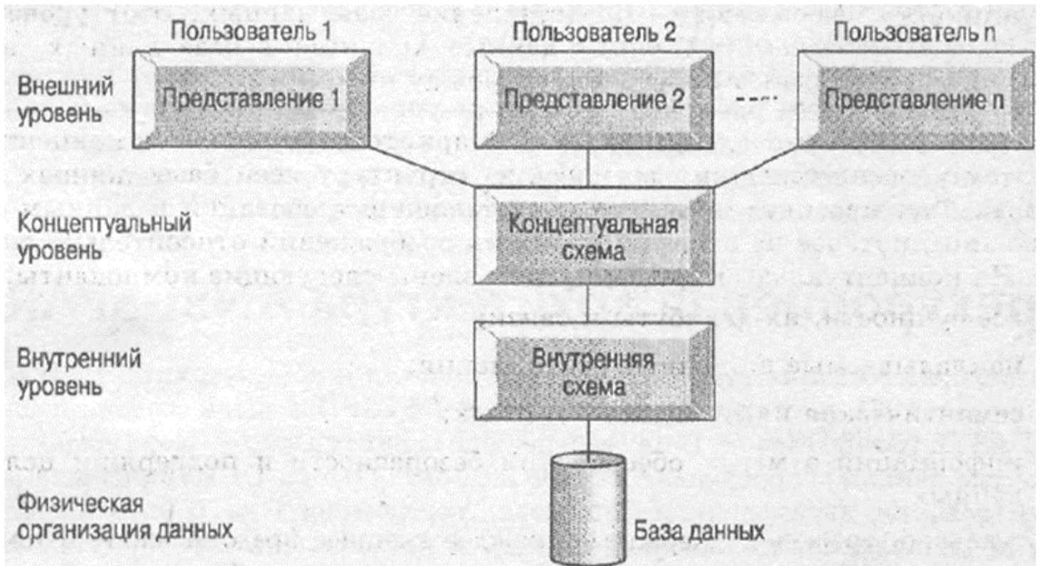
рисунок 1. Трехуровневая архитектура ANSI-SPARC.
